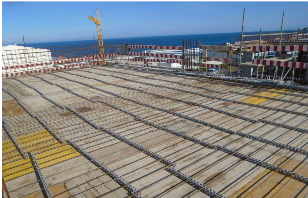
Fotografia 5 – Armaduras da Laje de Cobertura – Bloco A
