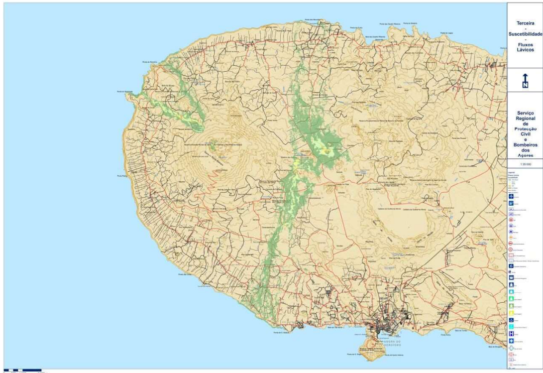
Figura 1 - Suscetibilidade Fluxos Lávicos
