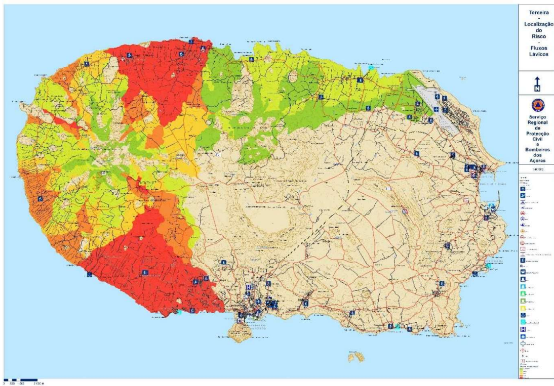
Figura 2 - Localização de Risco de Fluxos Lávicos
